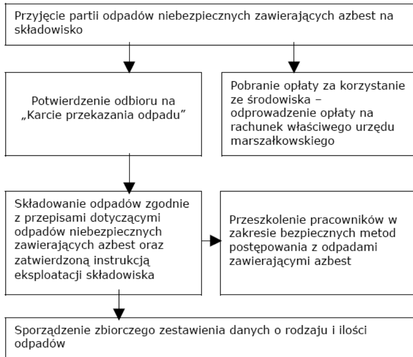
Rysunek 2 Schemat składowania odpadów azbestowych na składowisku odpadów Źródło: www.mgip.gov.pl
